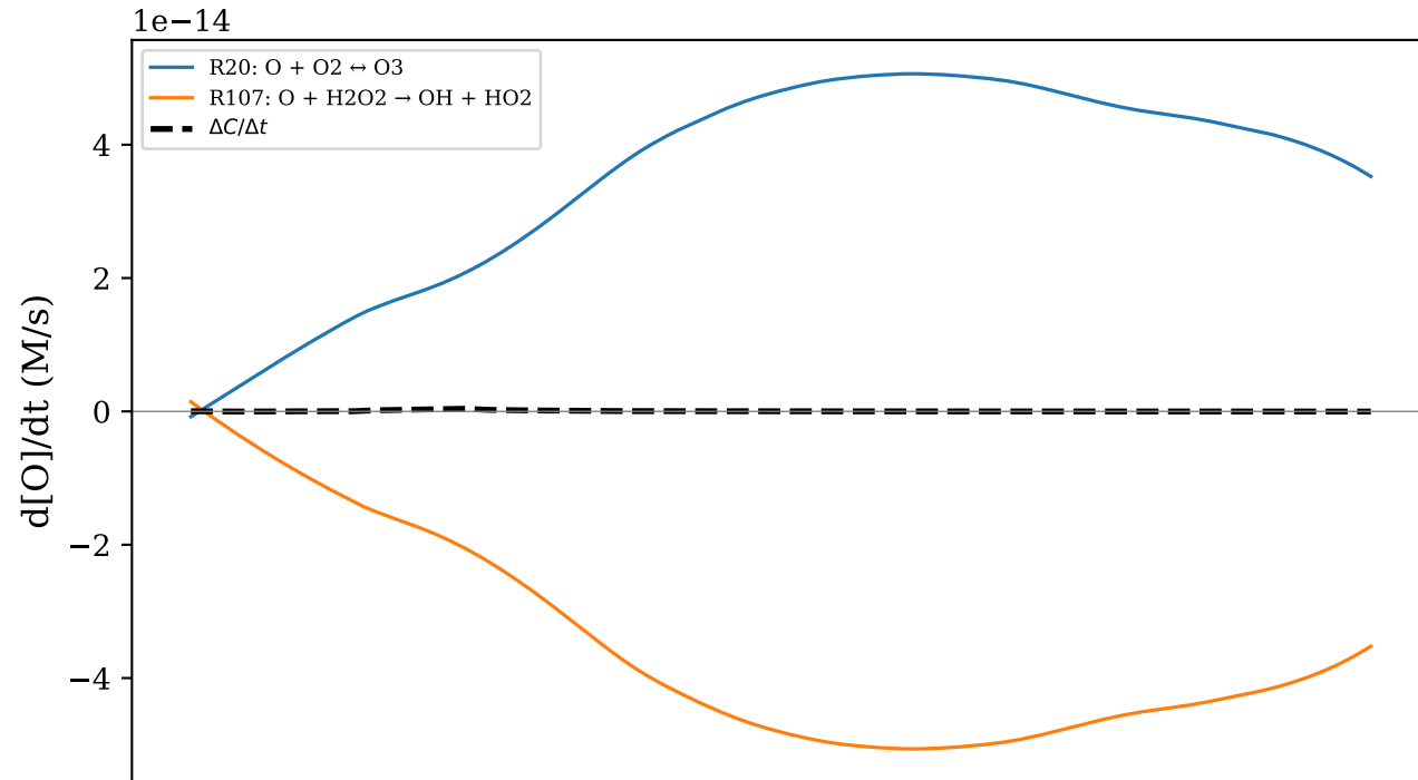
(a) O [final=-0.07 pM]
