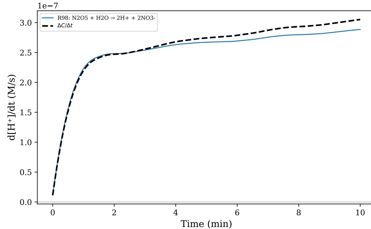
(d) H + [final=156.66 μM]
